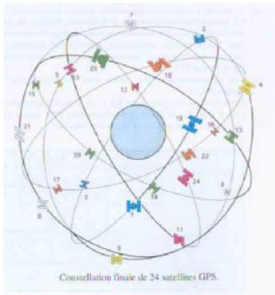
Constellation des satellites GPS
