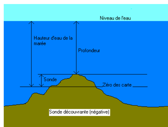
Sonde découvrante (négative)
